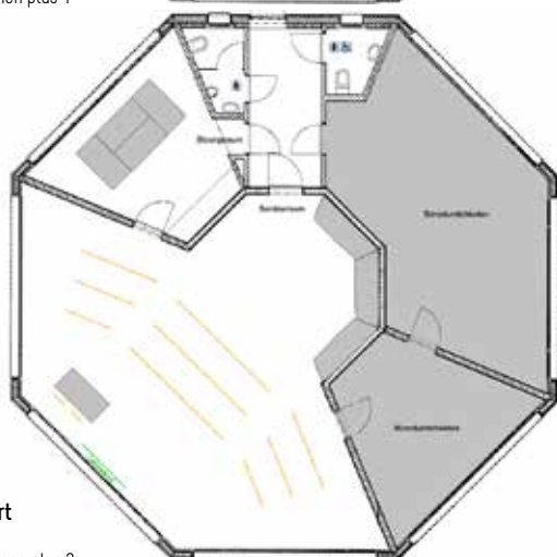
Hufeisen, klein
